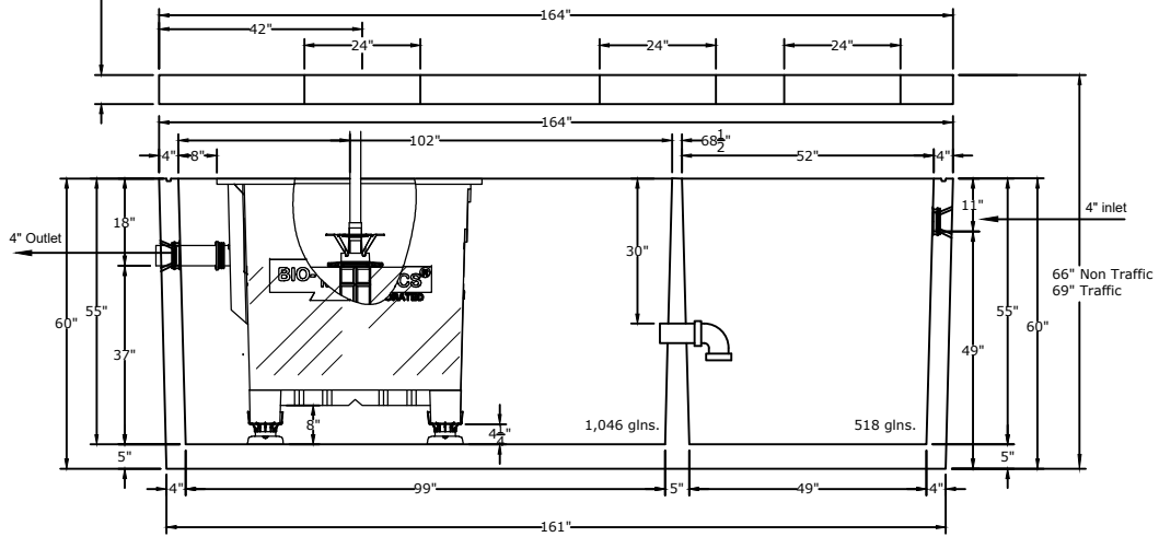
LONGITUDINAL SECTION
