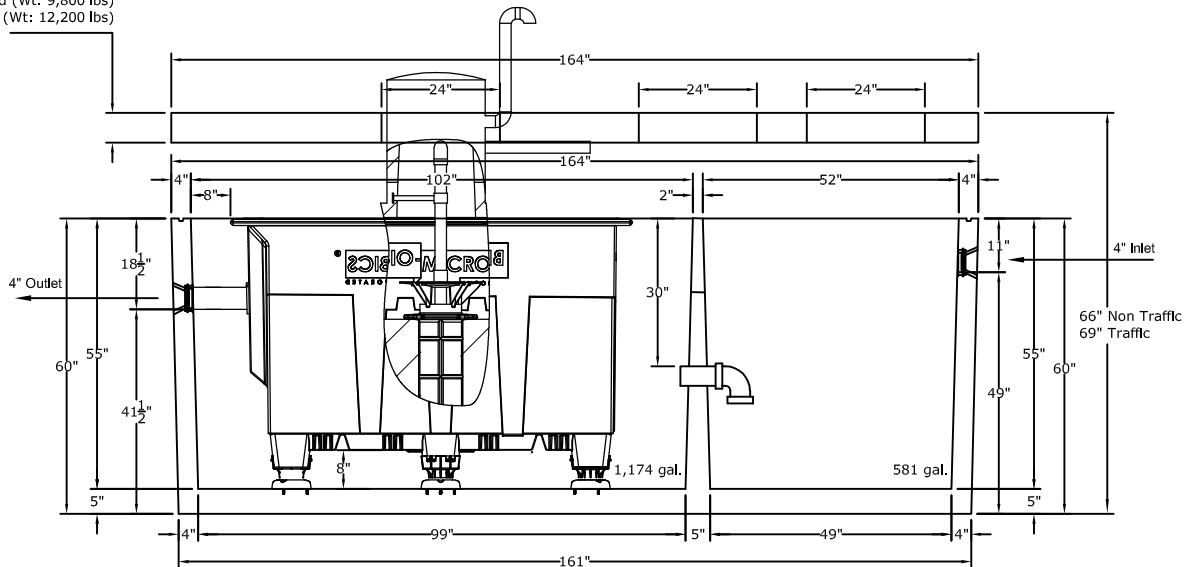
LONGITUDINAL SECTION
