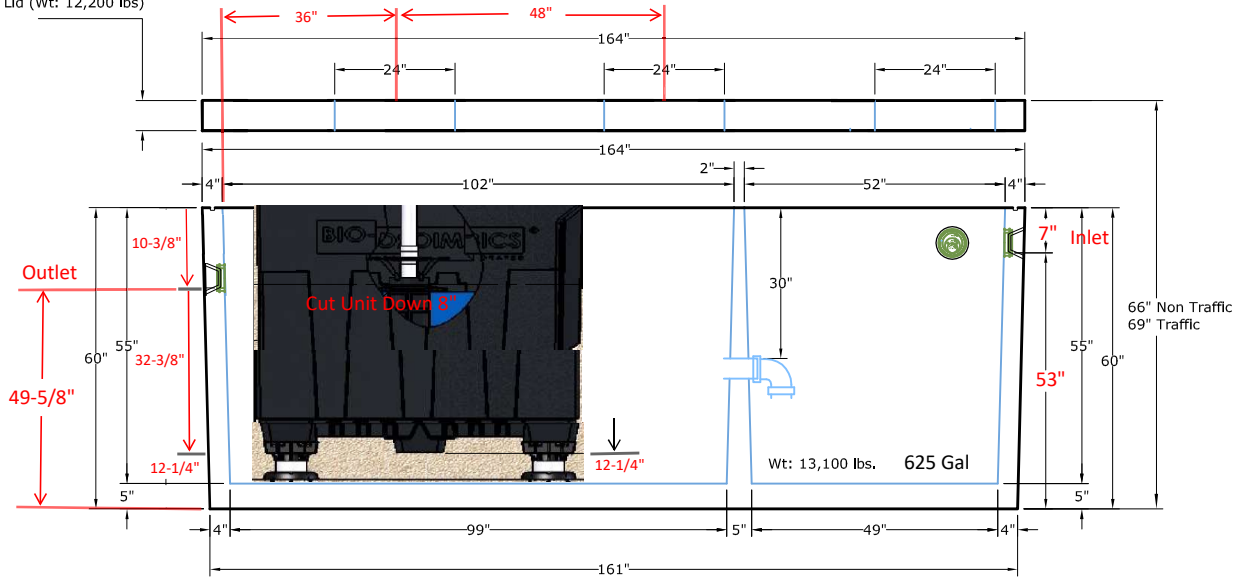
LONGITUDINAL SECTION
